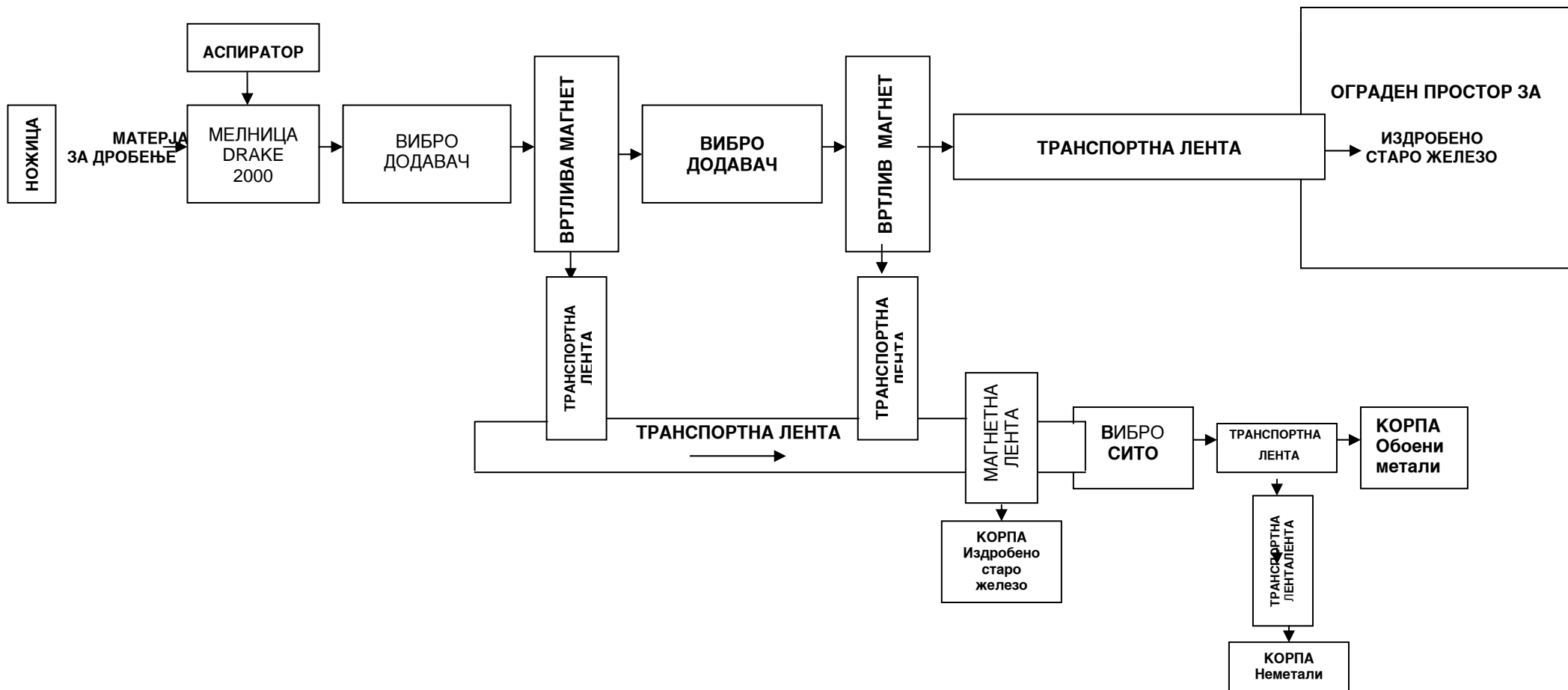
СЛ. 1 ШЕМАТСКИ ПРИКАЗ НА ПОСТРОЕЊЕТО ЗА ДРОБЕЊЕ НА СТАРО ЖЕЛЕЗО - ПРОИЗВОДСТВО НА ШРЕДЕР СО МЕЛНИЦАТА DRAKE 2000
