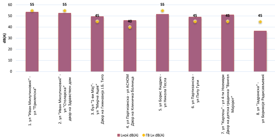
Графикон 4. Интензитет на бучава во животната средина во Битола за основниот индикатор Lн, 2023 година
