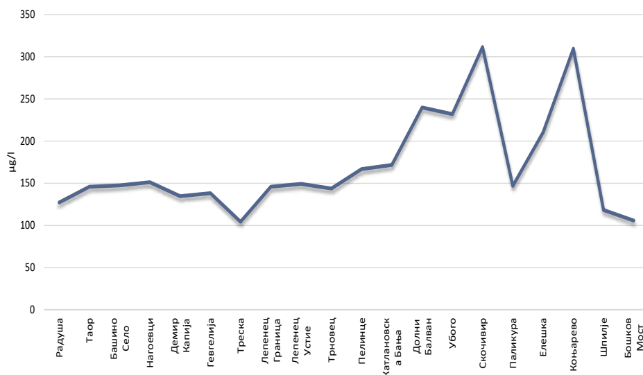
Графикон 1. Средногодишни концентрации на железо (Fe) во 2023 год
