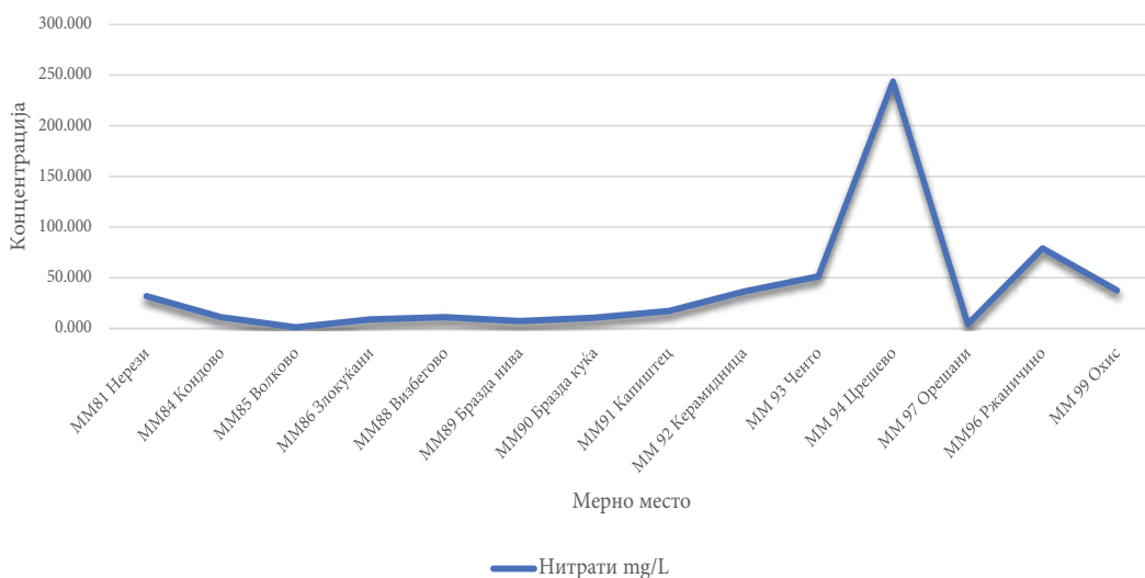
Графикон 7. Квалитет на подземни води во Скопската котлина и Град Скопје во 2023 година
