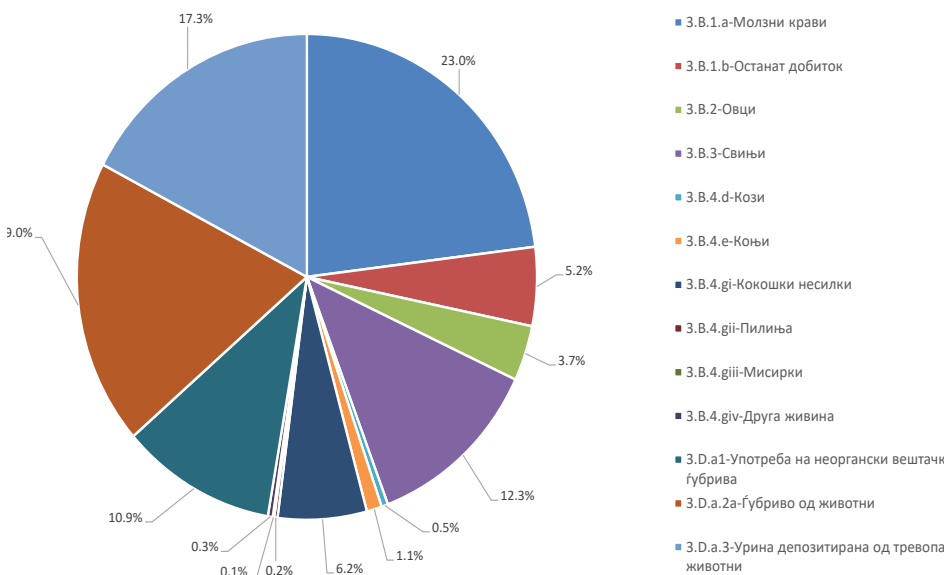
Графикон 27. Емисии на \text{NH}_3 од NFR категоријата Земјоделство по подкатегории во 2022 година
