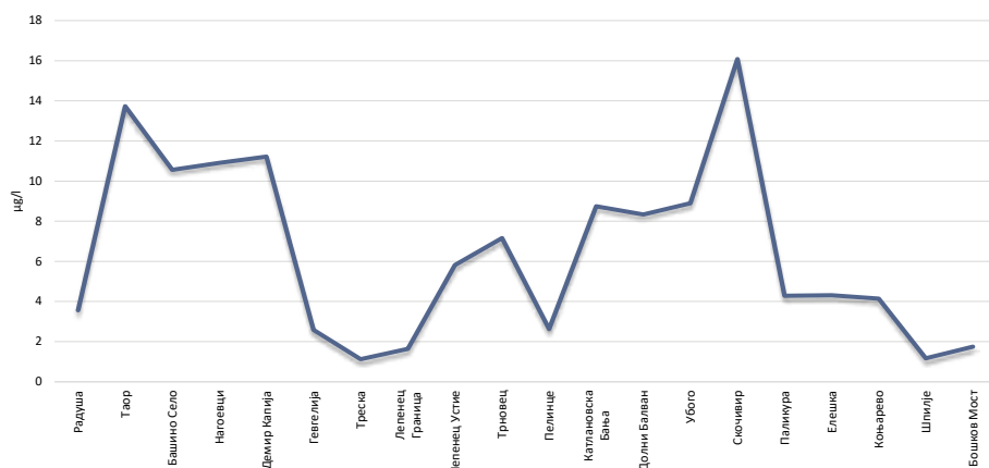
Графикон 3. Средногодишни концентрации на цинк (Zn) во 2023 год
