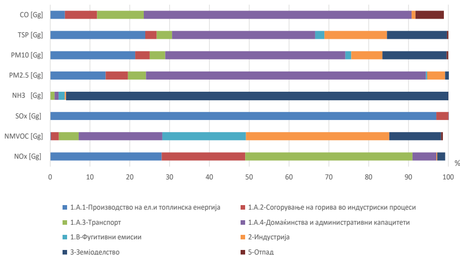
Графикон 2. Емисии на основните загадувачки супстанции и цврсти честички во 2022 година по NFR категории
