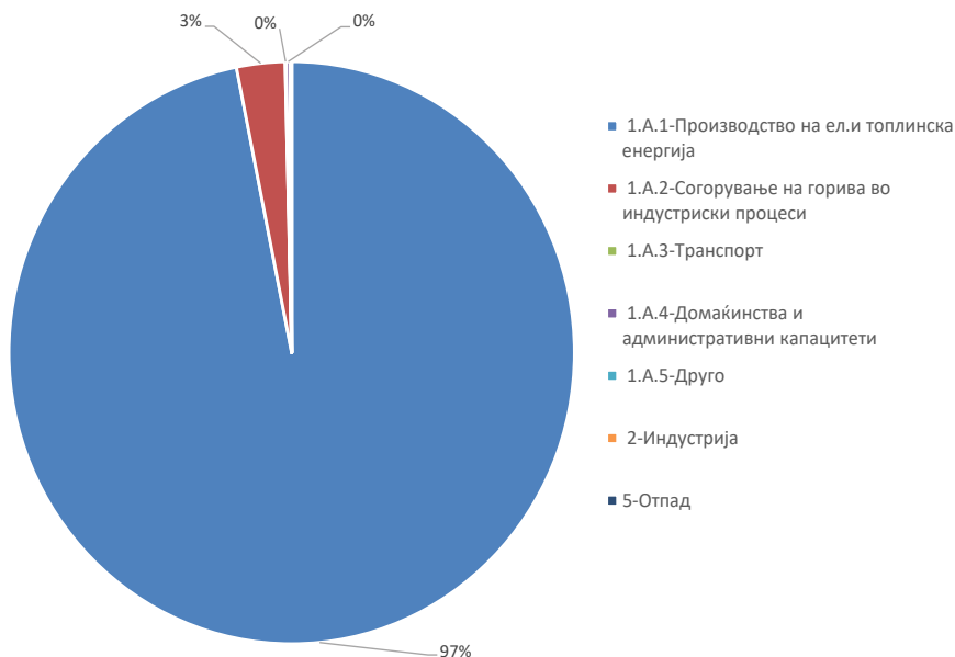
Графикон 7. Емисии на SO 2 во 2022 година по NFR категории
