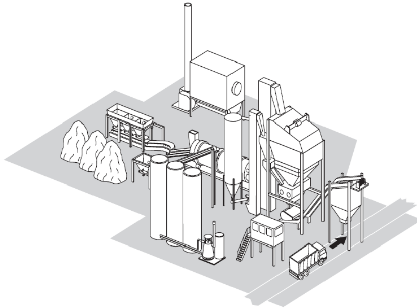
Слика 7. Составни делови на асфалтна база
