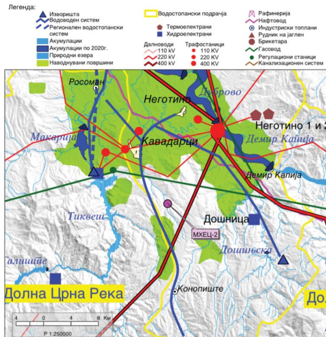
Слика 6: Водостопанска и енергетска инфраструктура
