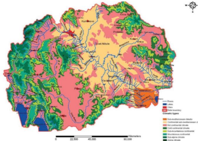
Слика 3: Климатски подрачја во Република Македонија
