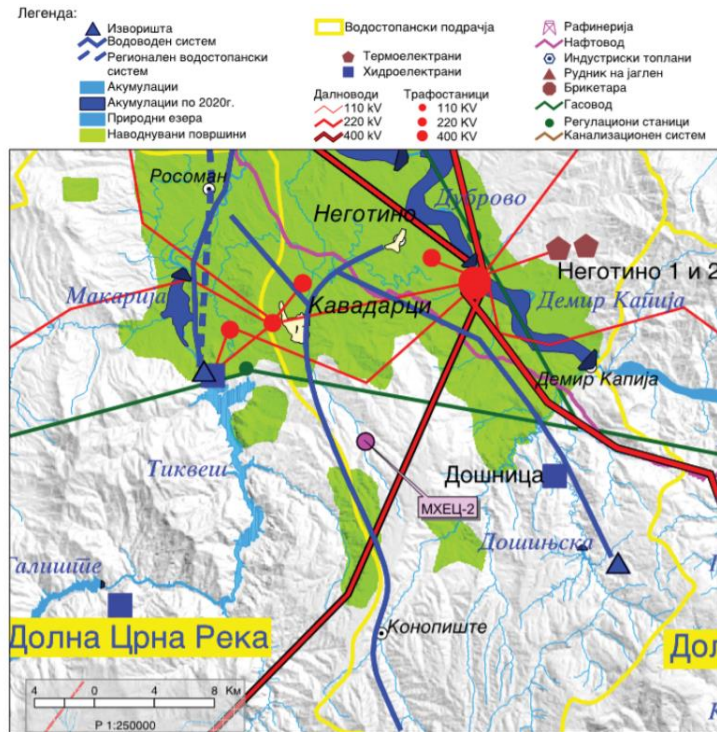
Слика 6: Водостопанска и енергетска инфраструктура
