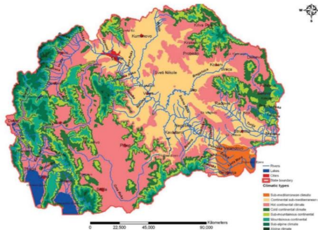
Слика 3: Климатски подрачја во Република Македонија
