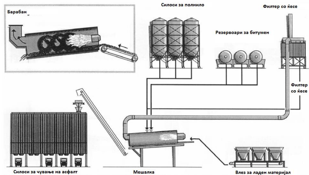
Слика 7 Шематски приказ на производството на асфалт
