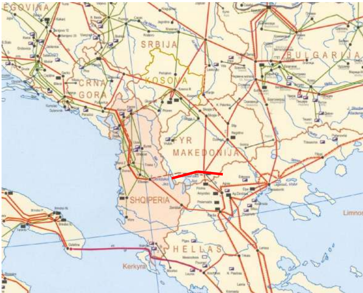
Планирана 400 kV интерконективна врска Битола(Македонија) – Елбасан(Албанија))
