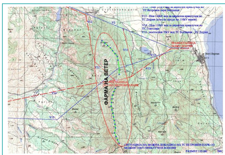
Слика бр.3: Парк на ветерни електрани со ТC 20/110kV и електроенергетски приклучок
